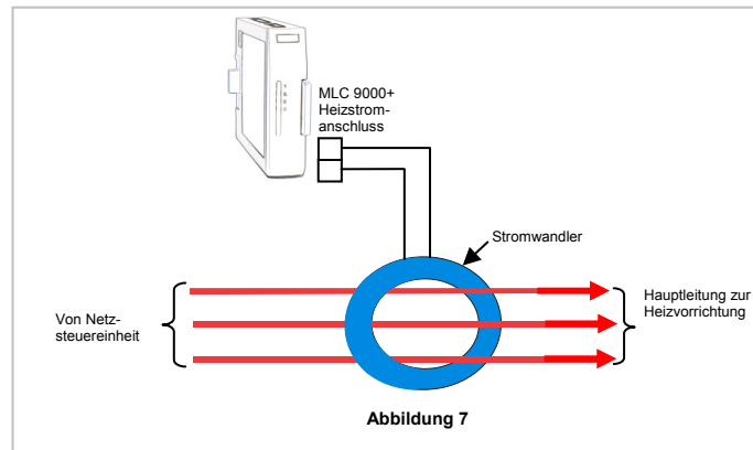
Abbildung 7 Beim örtlichen Händler erhältliche Stromwandler:
