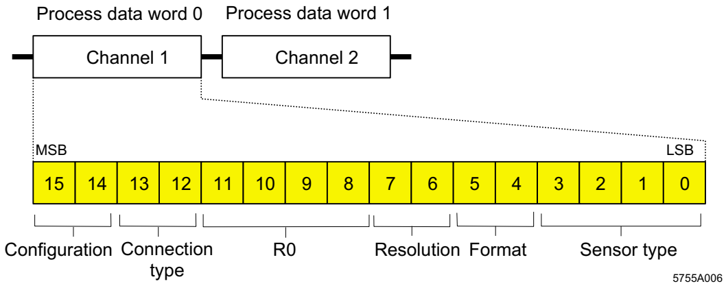
Bild 7 Process data output words
